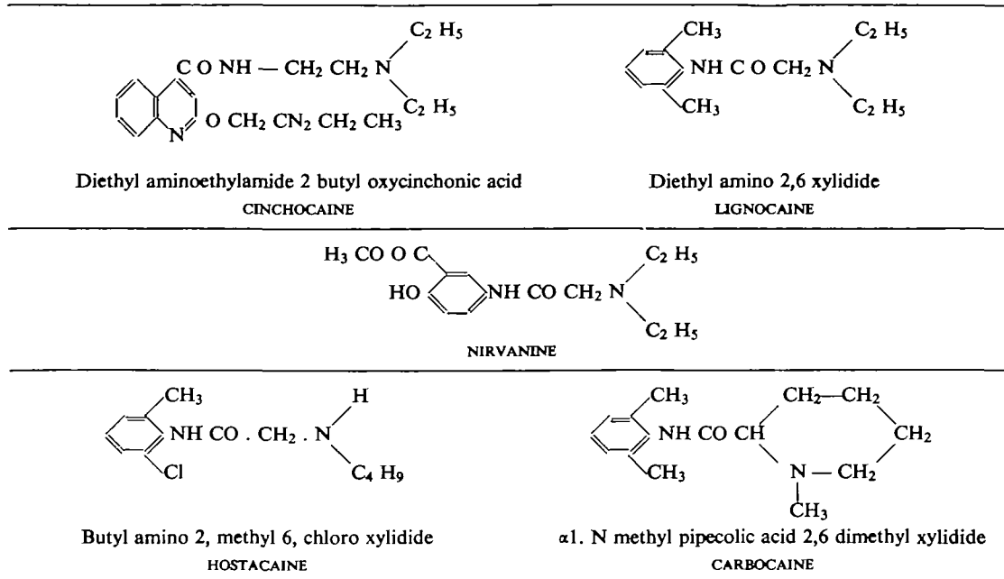
FIG. 8 Amides.
