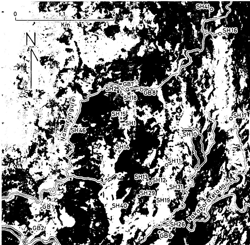
Fig. 4. Namurungule Sheet
