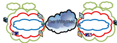
Fig. 6. VPN-extended VSN.
