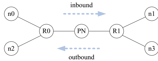
Fig. 8. A Tmix topology
