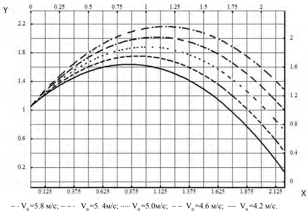
Рис.3. Графические характеристики траектории центра масс для различных значений начальной скорости вылета
