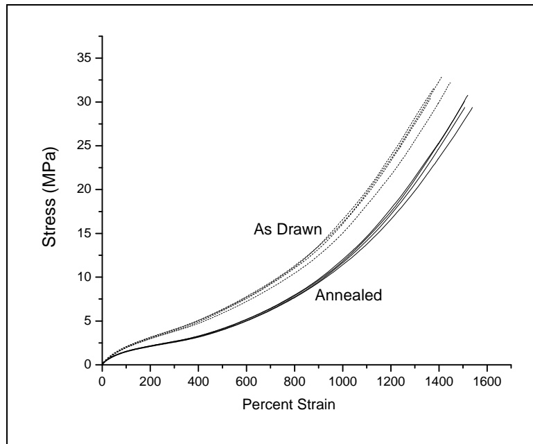
Figure 22. Tensile tests of IM 800A.
