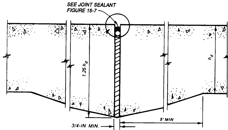
b. LONGITUDINAL
